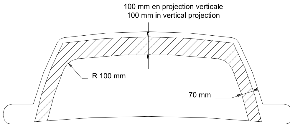
Mesures par rapport au bord de la surface vitrée 253-48
